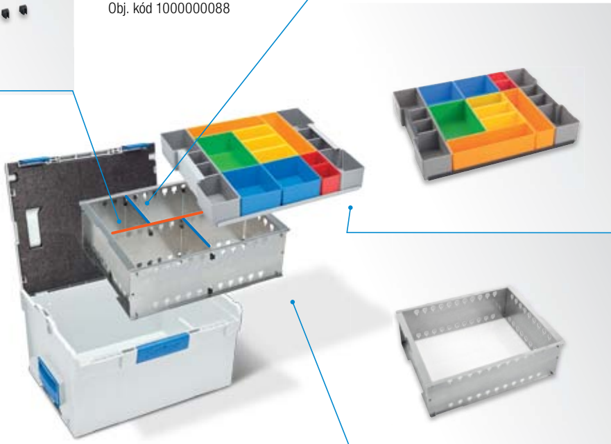
283 x 255 pro L-BOXX 374 LB 374 STB 283x255 Obj. kód 1000000088
